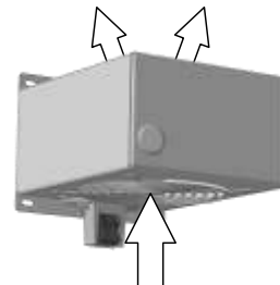
Рисунок 1. Рекомендованное монтажное положение
