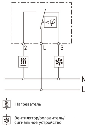
Схема подключения гигростатов MTN-410 и MTN-411
